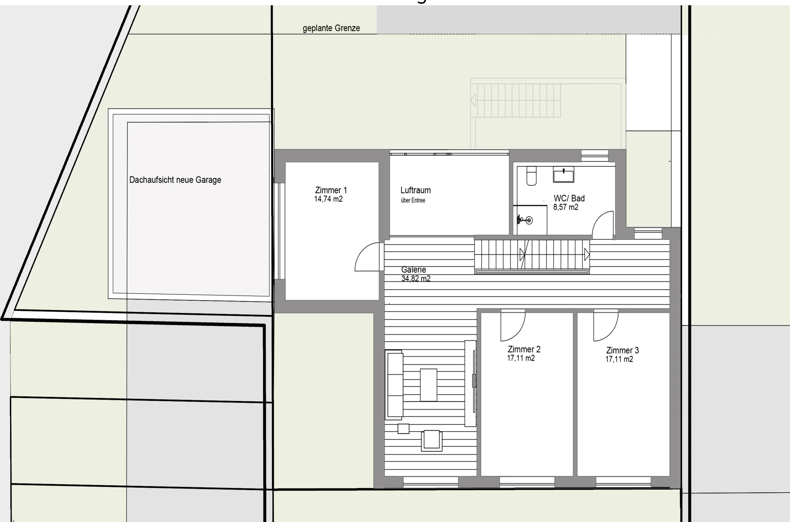
Grundriss Obergeschoss
