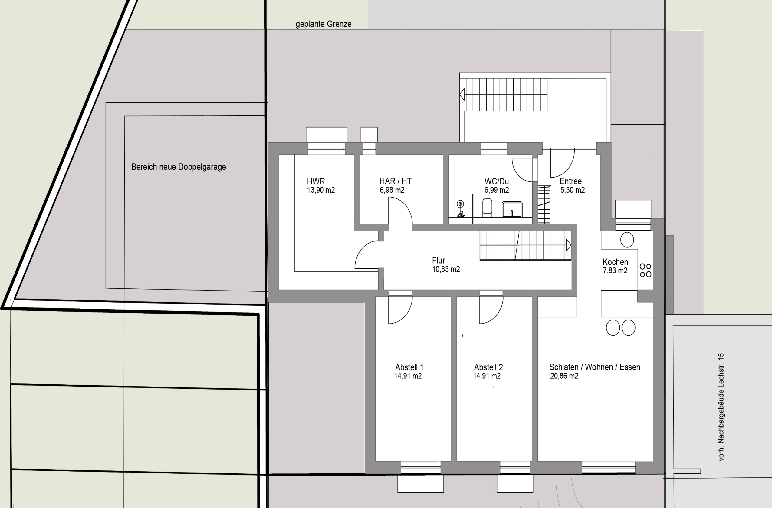
Grundriss Kellergeschoss
