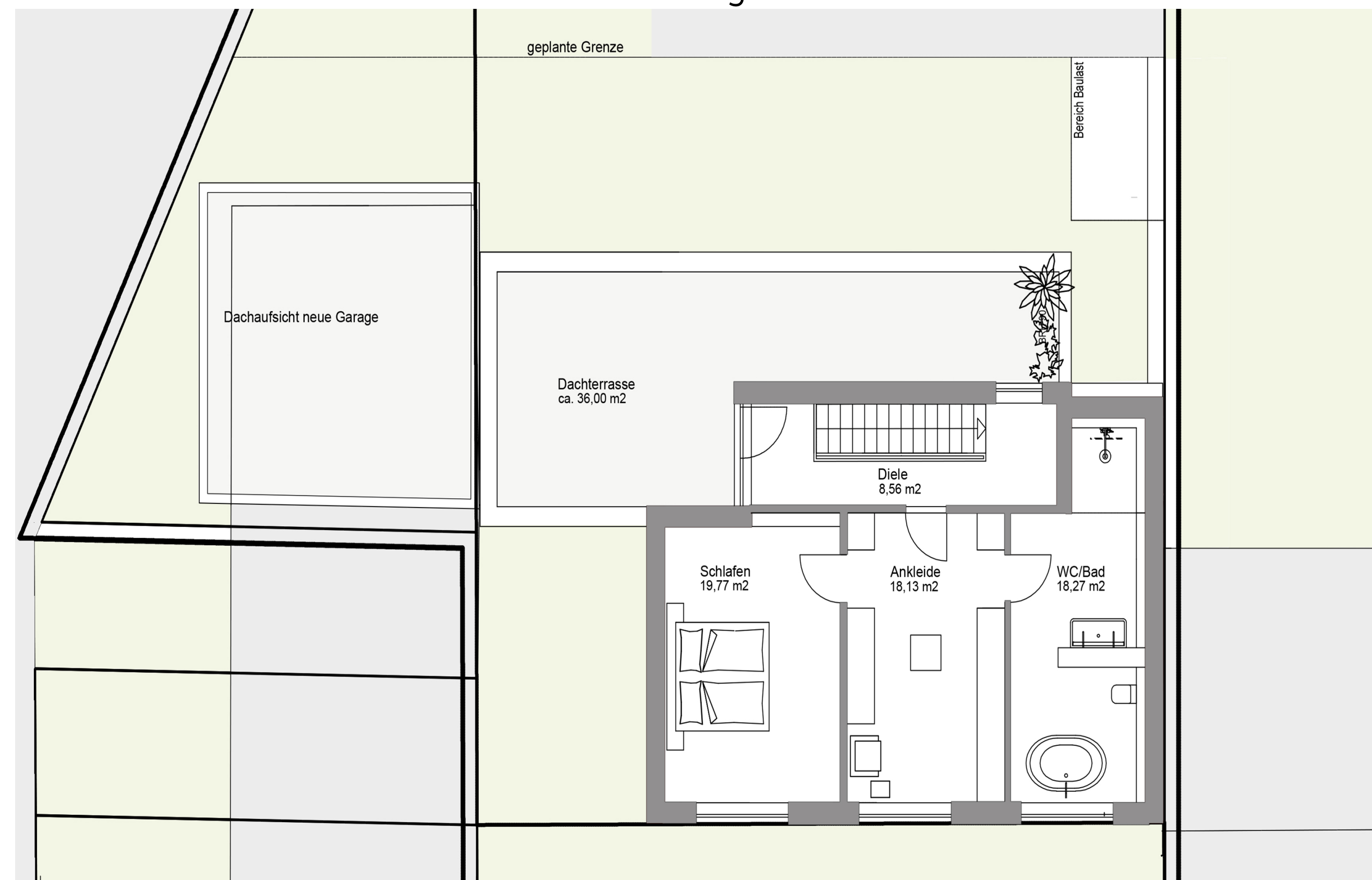
Grundriss Dachgeschoss
