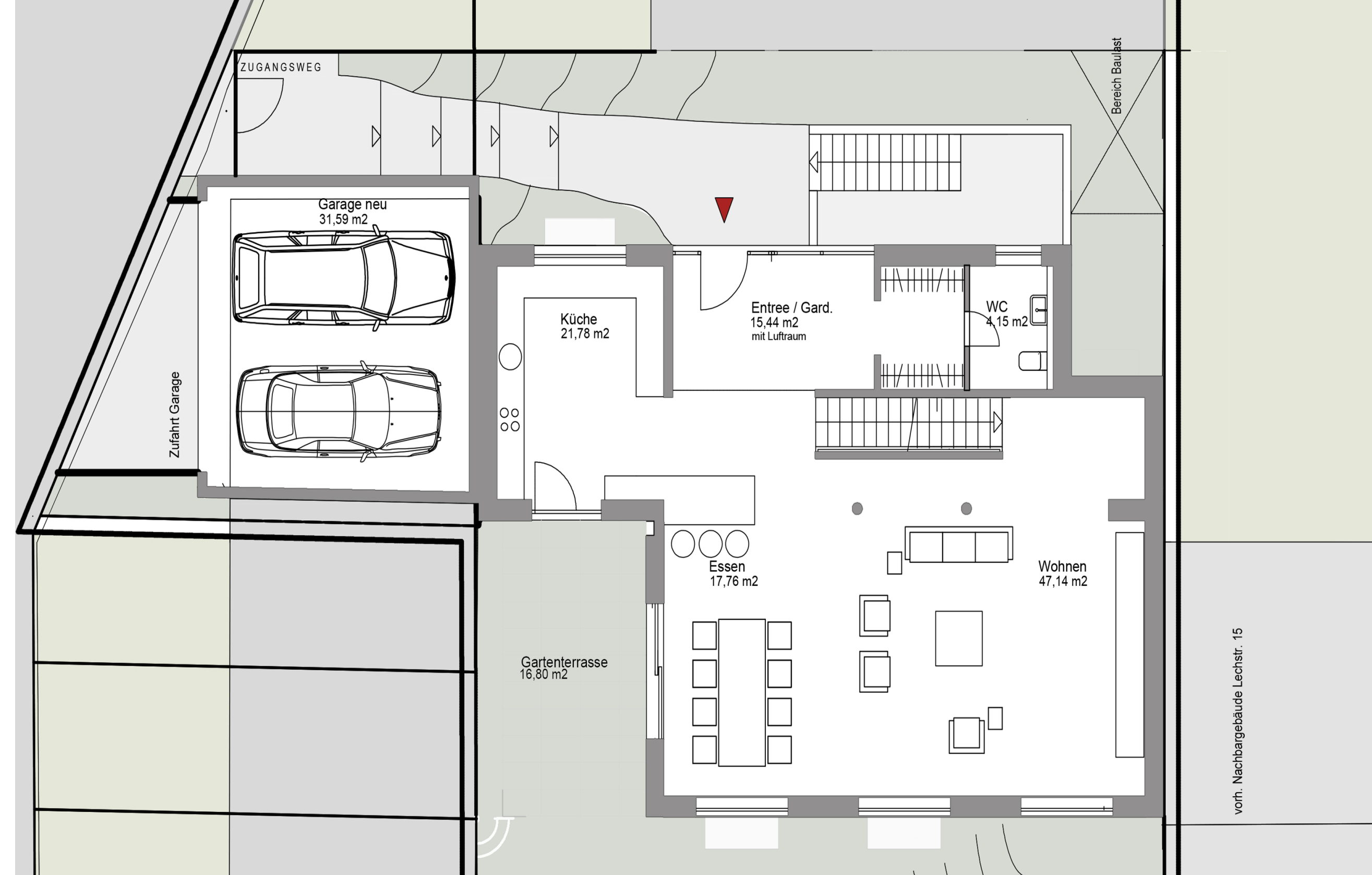
Grundriss Erdgeschoss
